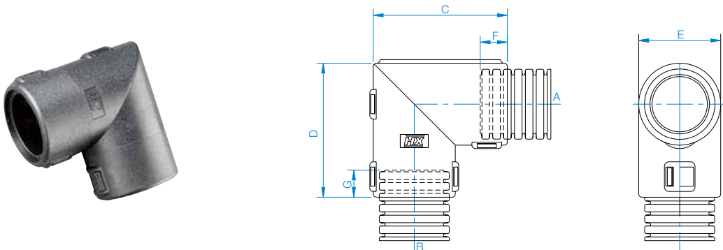
外部铰接肘型接头尺寸
