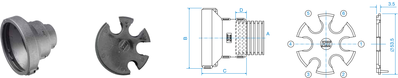
嵌入式圆形歧管尺寸
