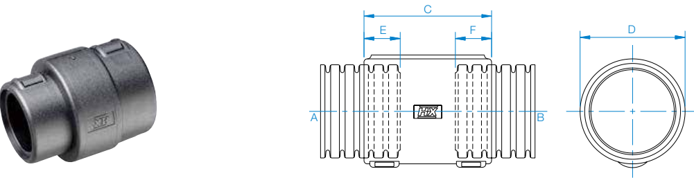
外部铰接结合头尺寸
